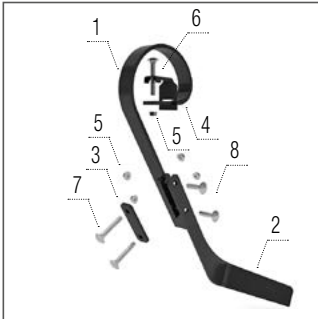
Deflector stânga
