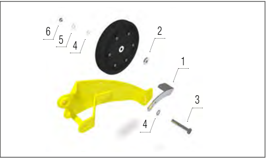
Răzuitor roată de adâncime Hardface
