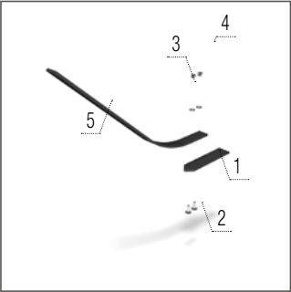
Răzuitor U-RING tăvălug
