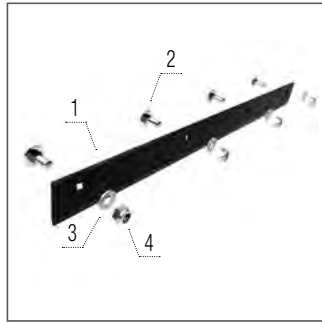
Lamă Trash Cutter 750
