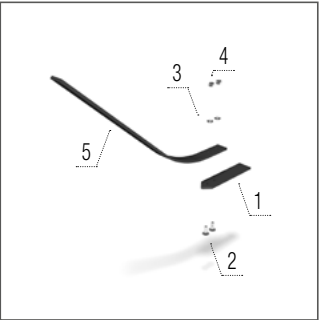
Răzuitor tăvălug cu arc
