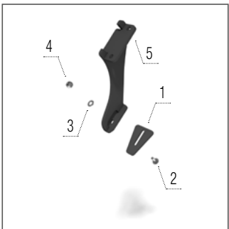
Răzuitor tăvălug Rubber
