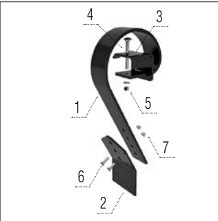
Suport pentru bara de nivelare
