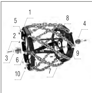
Tăvălug cu lanț 350
