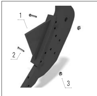
Spargător de brazdă M
