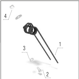
Dinte 6,3 mm
