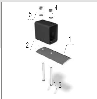
Contracuțițe în față
