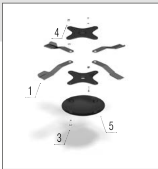
Lame pentru iarbă – stânga + capac rotor
