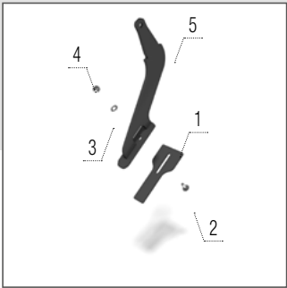
Răzuitor tăvălug Segment
