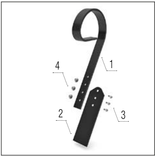
Suport pentru bara de nivelarea
