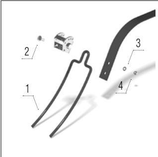
Dinte de grapă după brăzdar de semănat
