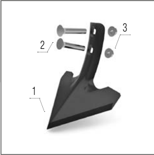
Săgeată 200 mm
