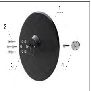
Brăzdar de semănat
