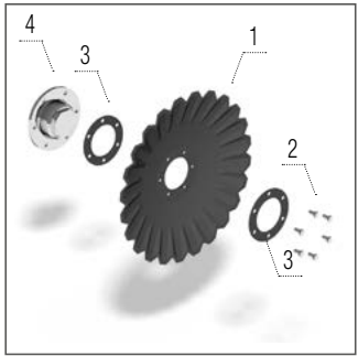
Disc A pentru unitatea centrală 620 × 6 mm
