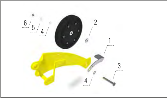
Răzuitor roată de adâncime clasică
