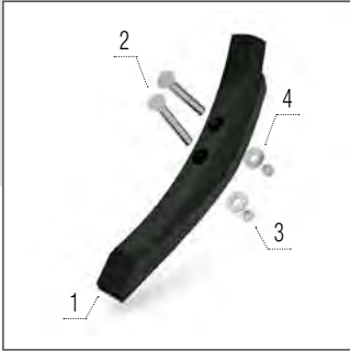
Daltă 50 mm LONG LIFE
