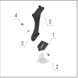
Răzuitor Cutpack
