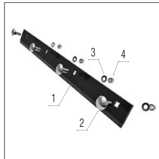
Lamă Trash Cutter 610
