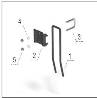
Dinte de grapă după tăvălug dublu
