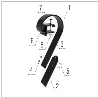
Suport pentru bara de nivelare în fața tăvălugului unic
