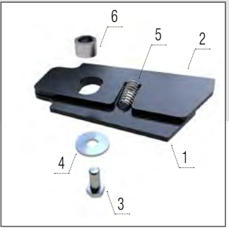
Răzuitor
