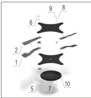
Lame pentru porumb – stânga + capac rotor
