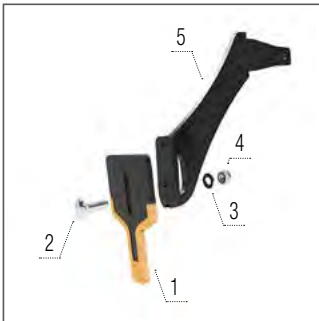
Răzuitor Cutpack Hardface
