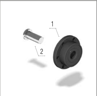
Lagăr brăzdar de semănat
