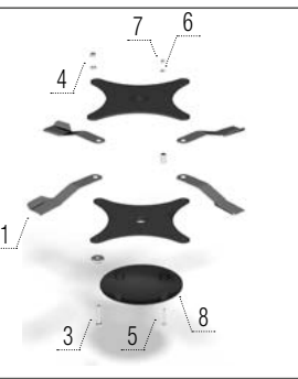
Lame pentru iarbă – stânga + capac rotor
