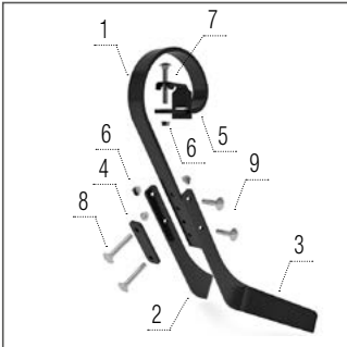
Deflector dublu
