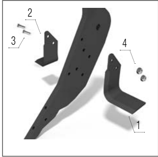
Aripă stânga și dreapta
