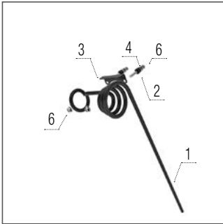
Dinte de grapă dreapta cu trei rânduri
