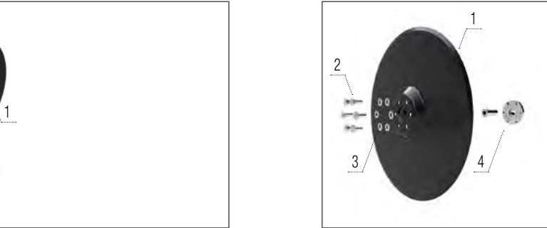
Roată de adâncime 330 × 65
