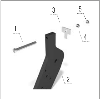
Șurub de forfecare D
