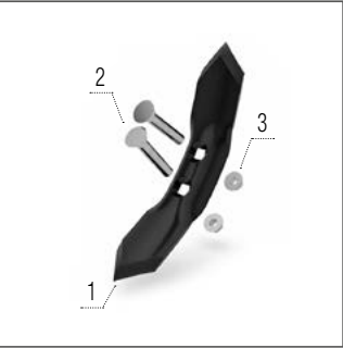
Daltă 60 mm
