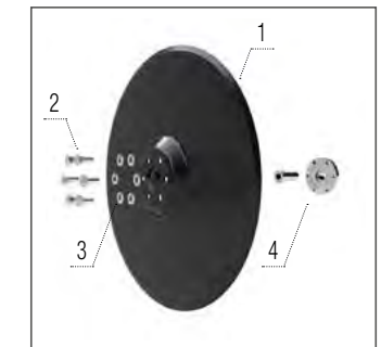
Brăzdar de semănat
