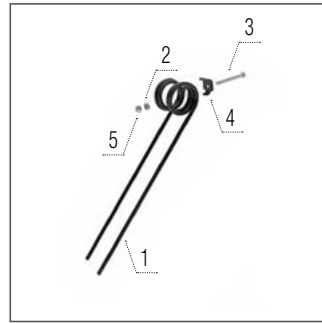
Dinte de grapă între discuri
