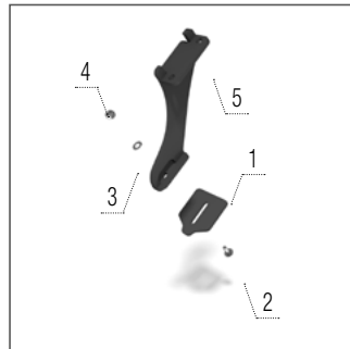
Răzuitor Cutpack
