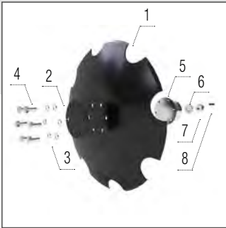
Disc zimțat 520 x 5 mm
