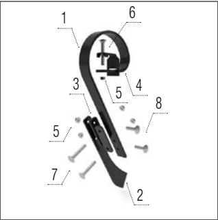
Deflector dreapta
