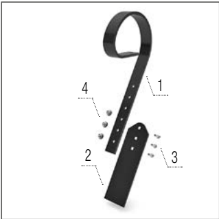
Suport pentru bara de nivelare sub brațul tăvălugului
