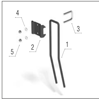
Dinte de grapă după tăvălug unic
