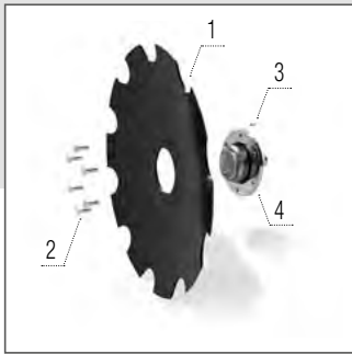
Disc zimțat pentru unitatea centrală 620 × 6 mm
