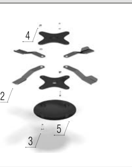
Lame pentru iarbă – dreapta + capac rotor
