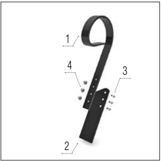
Suport central pentru bara de nivelare a tăvălugului
