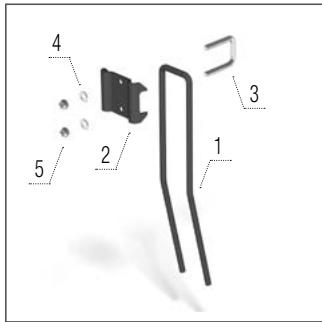
Dinte de grapă față
