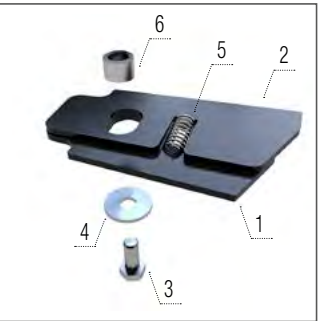
Răzuitor
