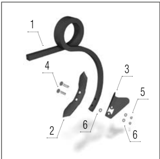
Daltă 60 mm
