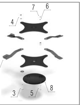
Fű kések – bal + rotor borítás
