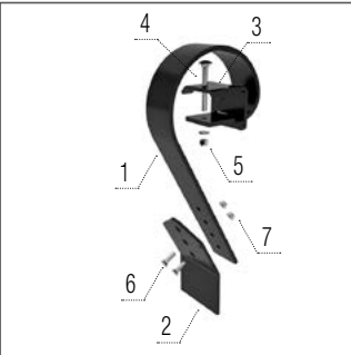
Crushbar simítólap előtt
