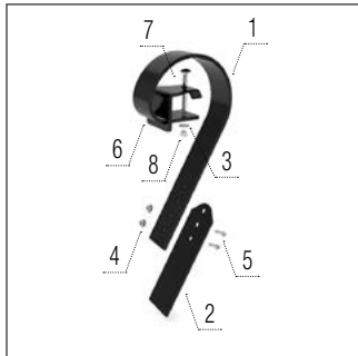
Simító lapát egysoros henger előtt
