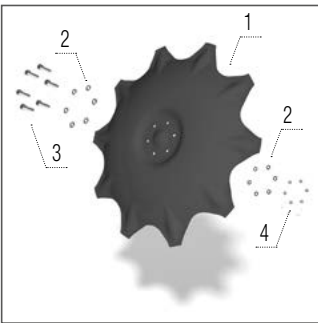
Védő tárcsa
