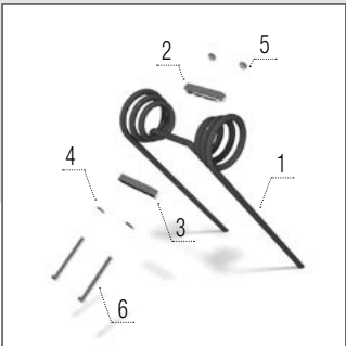
Pálca
