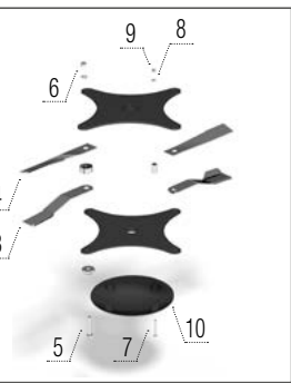
Kukorica kések – jobb + rotor borítás
