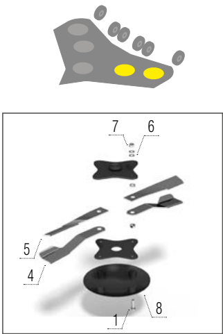
Kukorica kések – jobb + rotor borítás
