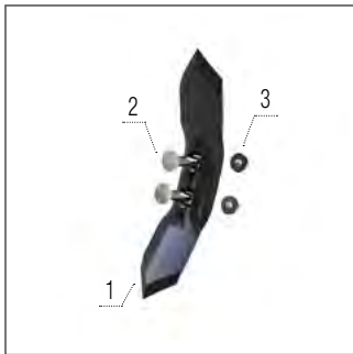
Nyomlazító kapa 1
