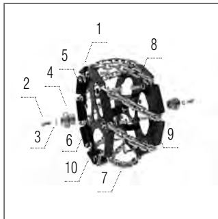
Láncos henger 200
