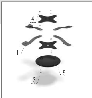
Fű kések – bal + rotor borítás
