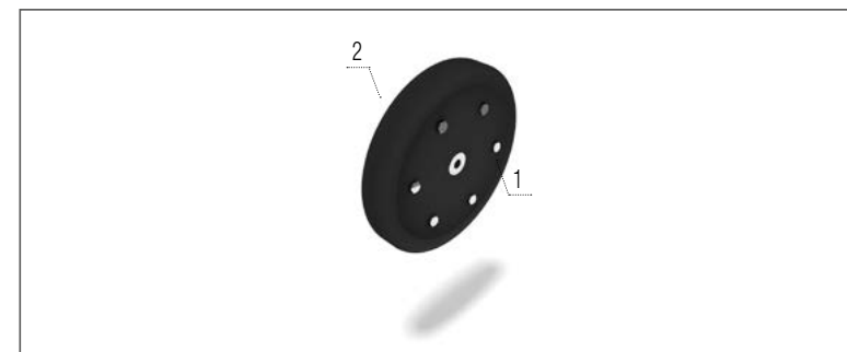
Nyomó kerék 330 × 50
