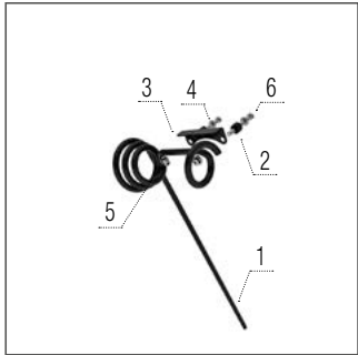
Három-soros baloldali borona pálca
