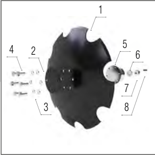
Csipkézett tárcsa 520 × 5 mm
