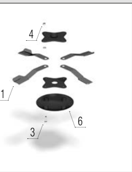
Fű kések – középső + rotor borítás
