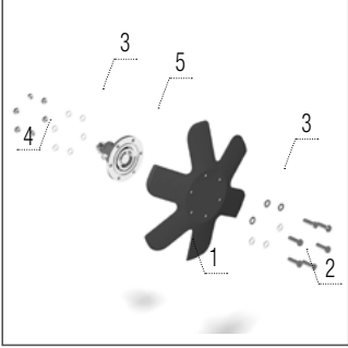
Egyengető csillag tárcsa – bal
