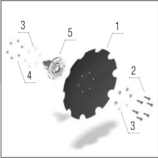
Csipkézett tárcsa 660 × 6 mm
