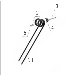
Borona pálca tárcsaszorok között
