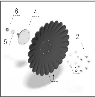
A-tárcsa 620 × 6 mm
