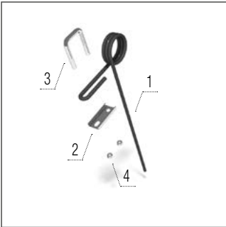
Borona pálca
