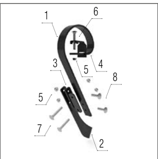
Jobb simító
