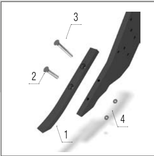
Kés 40 mm
