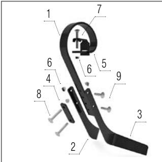
Dupla somító
