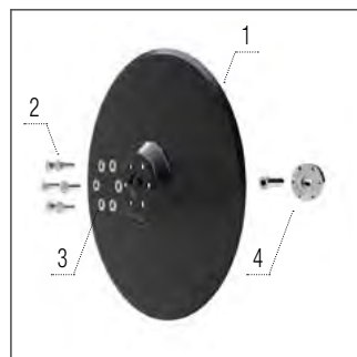
Vetőcsoroszlya
