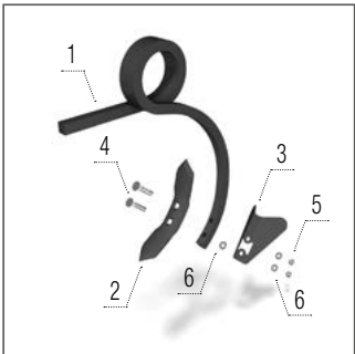
Kés 60 mm
