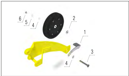
Klasszikus nyomókerék sárkaparó
