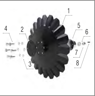
A-tárcsa 520 × 5 mm
