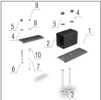
Melső ellenkés
