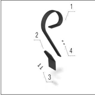
Crushbar simítólap – hátsó simító
