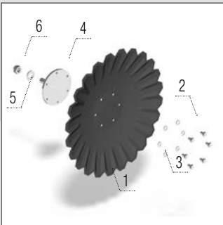
A-tárcsa 620 × 6 mm
