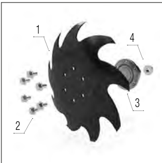
9-RH Csillag
