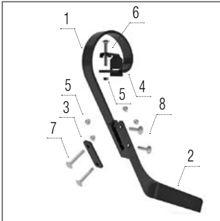
Bal simító
