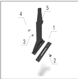
V-ring henger sárkaparó
