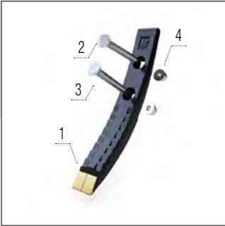
Kés 40 mm LONG LIFE
