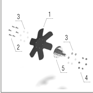
Egyengető csillag tárcsa – jobb
