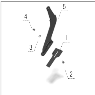
Szegmentált henger sárkaparó
