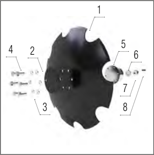
Csipkézett tárcsa 560 × 5 mm
