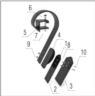
Crushbar simítólap után
