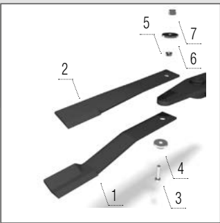
Kés
