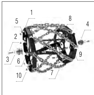
Láncos henger 350
