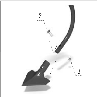
Kapa 150 mm
