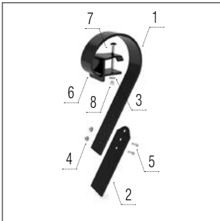
Simító lapát dupla henger előtt
