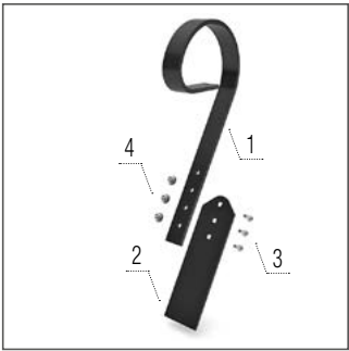
Hátsó hengerek előtti simító
