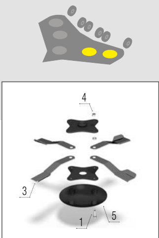
Fű kések – jobb + rotor borítás
