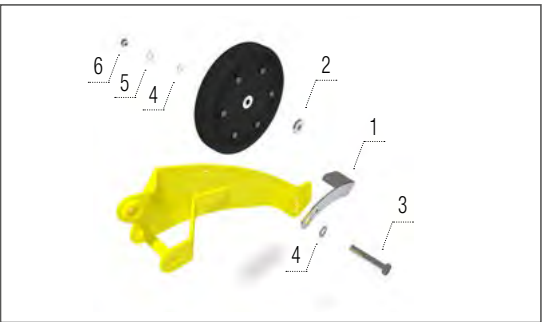
Hardface nyomókerék sárkaparó
