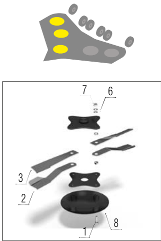
Kukorica kések – bal + rotor borítás
