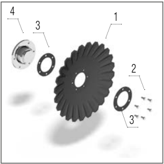
A-tárcsa a középső egységhez 620 × 6 mm
