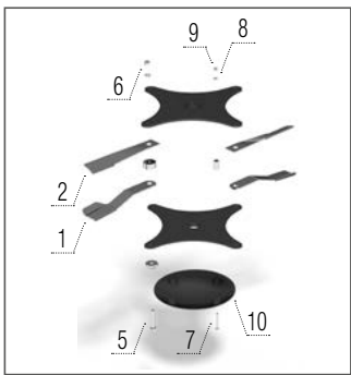
Kukorica kések – bal + rotor borítás
