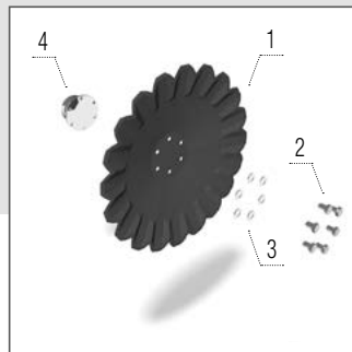
A-tárcsa 520 × 5 mm
