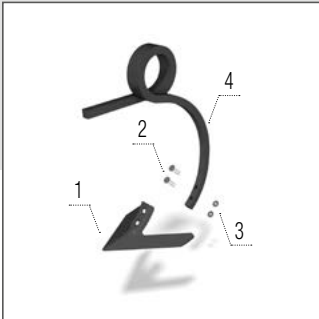
Kapa – jobb
