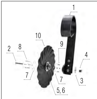
Csoroszlya – jobb
