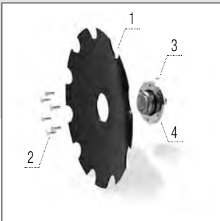
Csipkézett tárcsa a középső egységhez 620 × 6 mm
