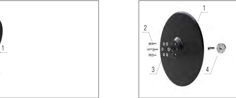
Nyomó kerék 330 × 65
