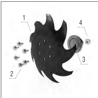
9-LH Csillag
