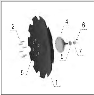
Csipkézett tárcsa 620 × 6 mm
