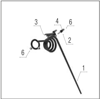
Három-soros jobboldali borona pálca
