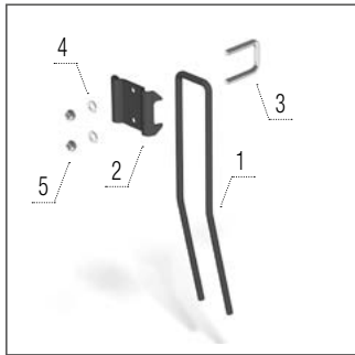
Melső borona pálca
