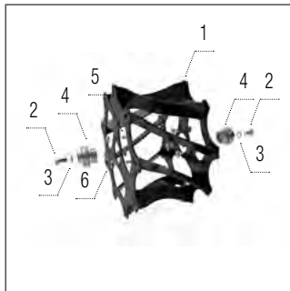
Pálcás henger 200
