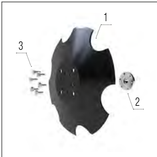
Marqueur de pré-levée
