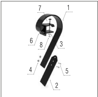
Bande niveleuse devant un double rouleau
