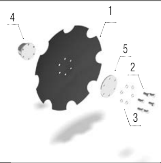
Disque crénelé 520 × 5 mm
