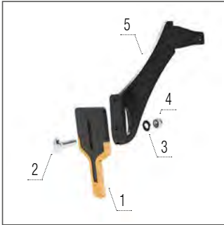
Décrotteur de rouleau Hardface Cutpack
