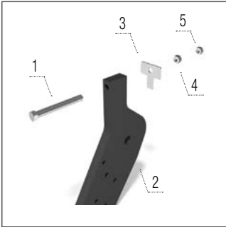
Boulon de sécurité D
