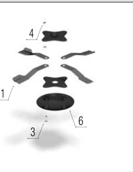
Couteaux à herbe – centraux + coupole
