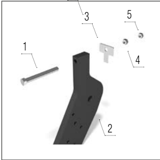
Boulon de sécurité M
