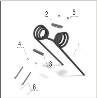
Peigne de travail
