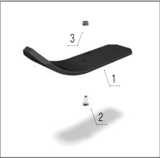
Pâtins de protection
