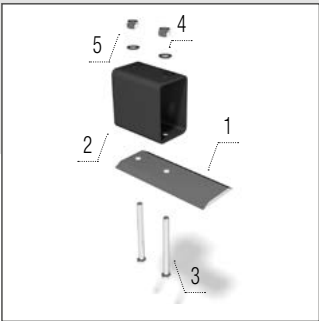
Contre couteau avant
