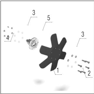
Disque étoile – gauche
