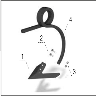
Soc – droit
