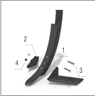
Ailettes de pointes 185 mm
