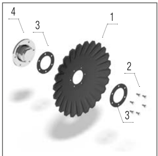
Disque A sur l'unité centrale 620 × 6 mm
