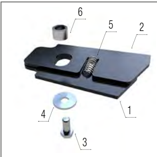
Décrotteur à couteaux
