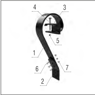
Niveleur Crushbar avant
