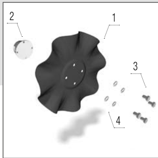
Disque PROFI
