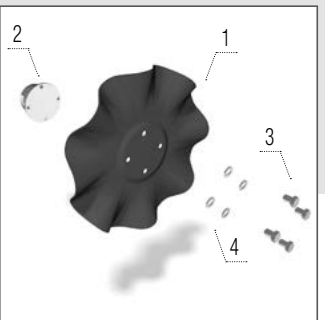
Disque PROFI
