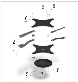
Couteaux à maïs – gauches + coupole
