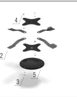
Couteaux à herbe – droits + coupole
