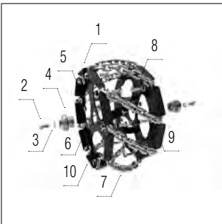
Rouleau à chaînes 200
