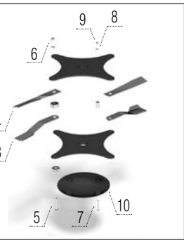
Couteaux à maïs – droits + coupole
