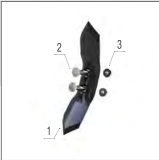
Efface traces 1 Modèle CS 1 – KM060324 POINTE..... 1 pièce 2 – KM000857 VIS ..... 2 pièce 3 – KM000296 ÉCROU ..... 2 pièce
