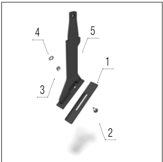
Décrotteur de rouleau U-Ring
