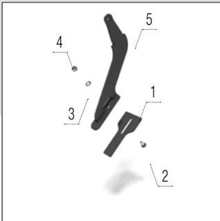
Décrotteur de rouleau à segments
