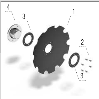
Disque crénelé sur l'unité centrale 620 × 6 mm
