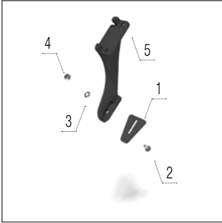
Décrotteur de rouleau Rubberpacker
