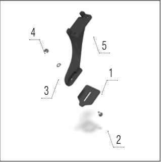
Décrotteur de rouleau Cutpack Rouleau
