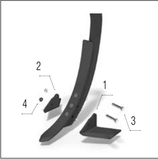
Ailettes de pointes 125 mm
