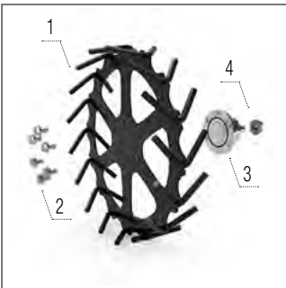
Rouleau à doigts 350 × 100
