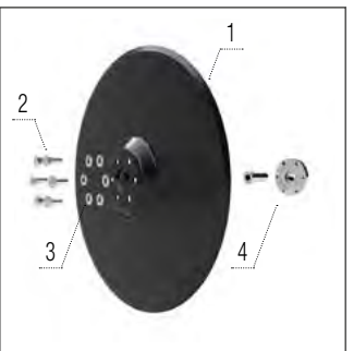
Disque de semis
