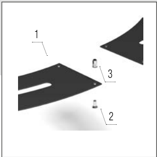
Kit de blindage
