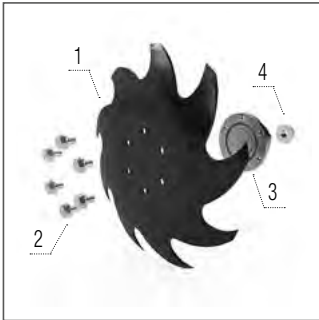
9-LH Étoile
