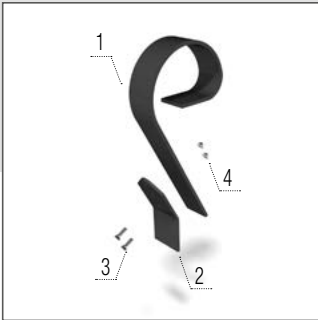
Niveleur Crushbar
