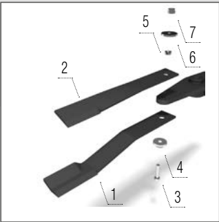
Couteau
