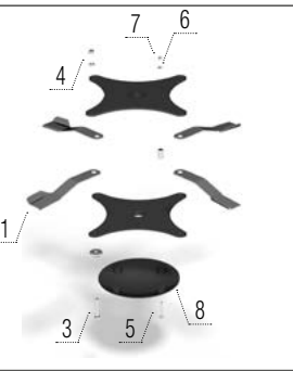
Couteaux à herbe – gauches + coupole
