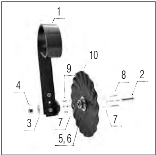
Disque TURBO – gauche
