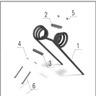
Peigne de travail – LONG LIFE
