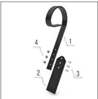
Cloison du rouleau
