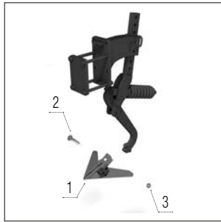
Soc d'efface-traces
