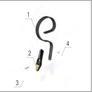
LONG LIFE Gamma tip
