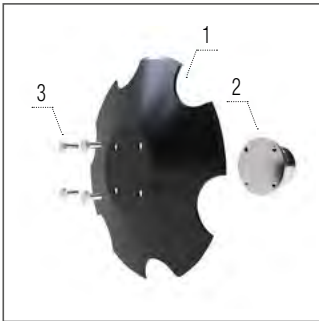
Seitliche Spuranreißer
