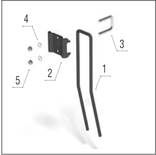
Striegel hinter einer einfachen Walze
