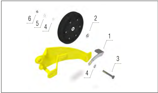
Abstreifer des Tiefenrads Hardface
