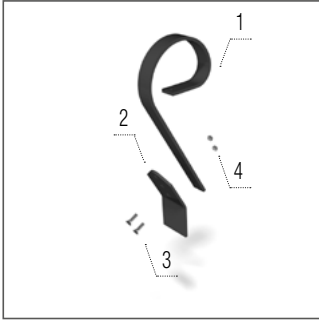
Streichschaufel Crushbar – hintere Planierschiene
