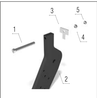
Ziehschraube M
