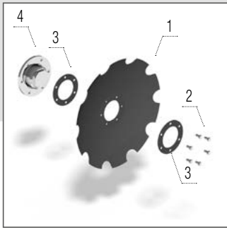
Gezahnte Scheibe auf der Mitteleinheit 620 × 6 mm
