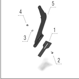
Abstreifer Segmentwalze
