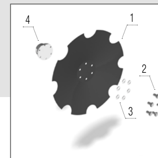
Gezähnte Scheibe 460 x 5 mm
