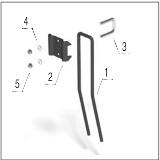
Striegel vor einer einfachen Walze
