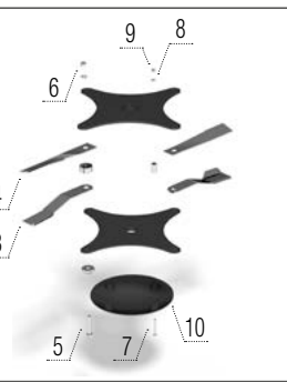
Maismesser – rechts + Rotorabdeckung
