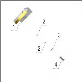
Abstreifer der Sähschabe Hartmetall
