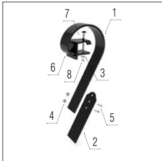
Planierschiene vor einer doppelten Walze
