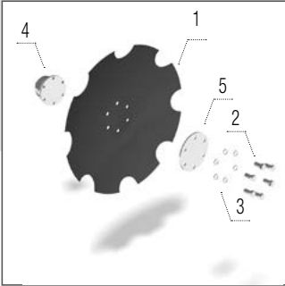
Gezahnte Scheibe 520 x 5 mm
