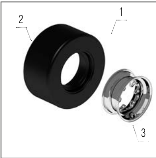
Heckbereifung
