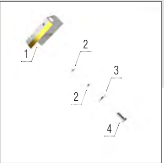
Abstreifer der Sähscheibe Hartmetall
