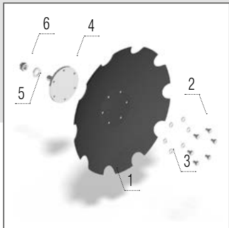
Gezahnte Scheibe 620 × 6 mm
