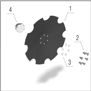
Gezahnte Scheibe 520 × 5 mm
