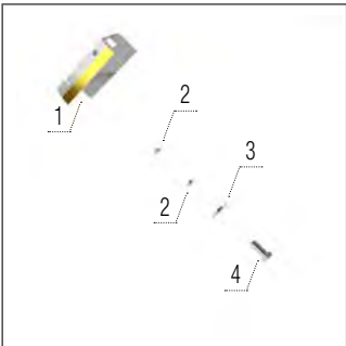
Abstreifer der Sähschleibe Hartmetall
