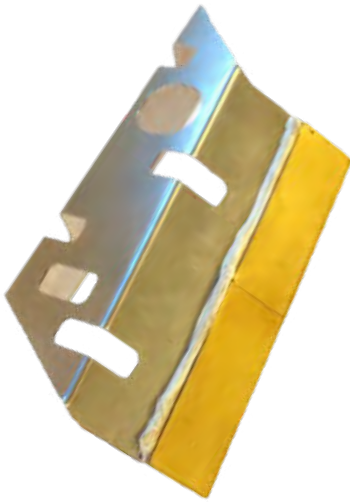
OMEGA OO_L, OO_FL KM060563 Abstreifer der Sähscheibe (1 St.)
