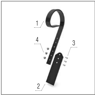
Packerblende unter dem Packerrahmen
