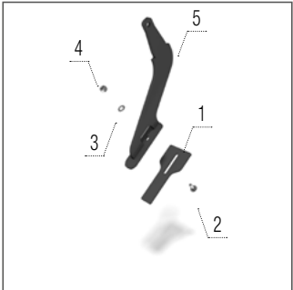
Abstreifer Segmentwalze
