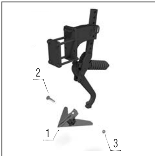
Zinken des Spurlockers
