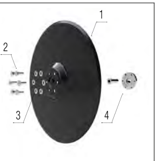
Disk na výsev
