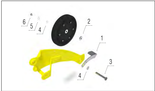
Stěrka hloubkového kolečka Classic
