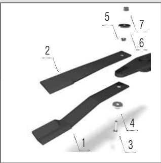
Nůž
