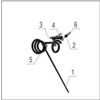
Zavlačovač třířadý levý
