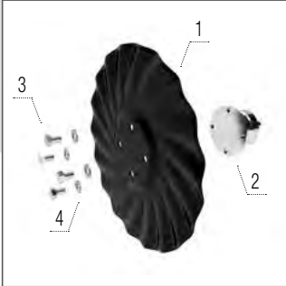
Turbocoulter pravý
