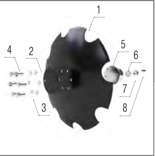
Zubatý disk 560 × 5 mm
