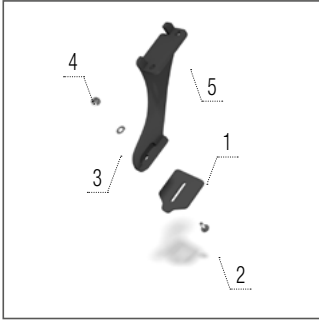
Stěrka Cutpack válec
