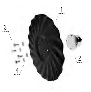
Turbocoulter levý
