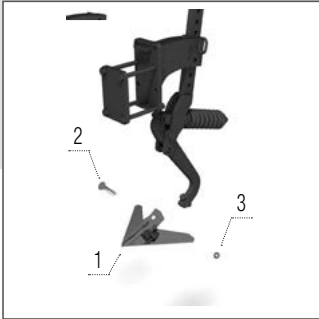
Radlička kypřiče stop traktoru
