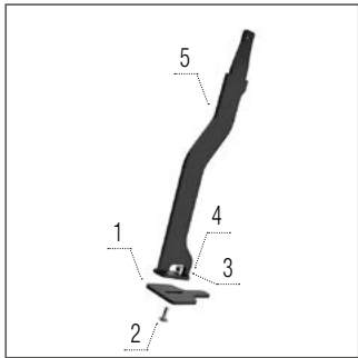
Stěrka Cutpack
