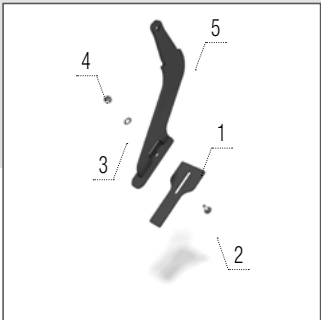
Stěrka Segmentový válec
