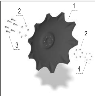
Ochranný disk
