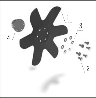
Rotační hvězdice – levá
