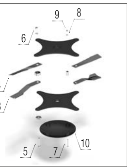
Nože kukuřičné – pravé + kryt rotoru
