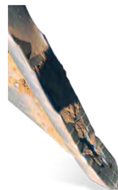
Dláto Long-Life po zpracování 700 ha půdy
