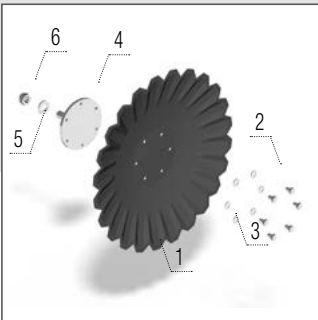
A-disk 620 × 6 mm
