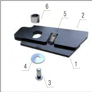
Nůžková stěrka
