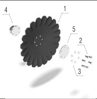
A-disk 520 × 5 mm
