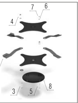
Nože travní – levé + kryt rotoru
