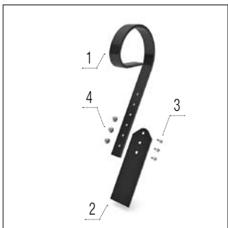
Clona pěchu pod ramenem pěchu
