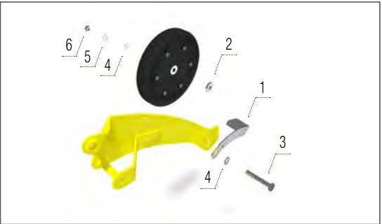
Stěrka hloubkového kolečka Hardface
