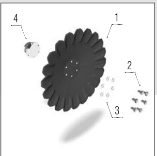
A-disk 520 × 5 mm
