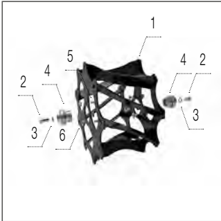
Решітчастий коток 200
