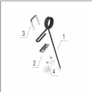
Стійка борони
