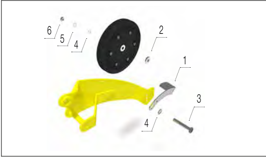
Скребок копіювального колеса з твердим наплавленням
