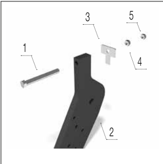
Стяжний болт D
