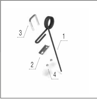
Стійка борони
