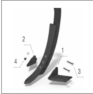
Крила долота 125 мм
