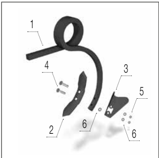
Долото 60 мм
