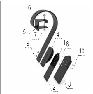
Планка Crushbar – задній вирівнювач
