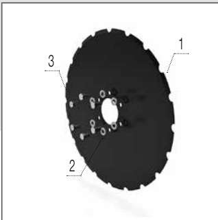
Зубчастий диск 508×5
