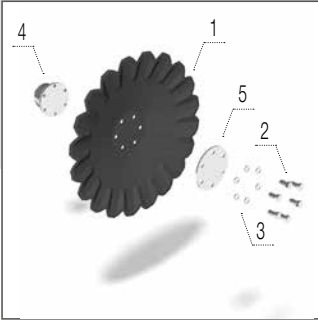
А-диск 520 × 5 мм
