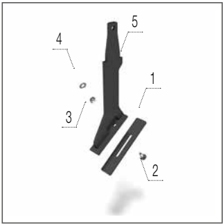
Скребок V-подібного кільцевого котка
