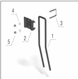
Передня стійка борони
