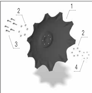
Захисний диск
