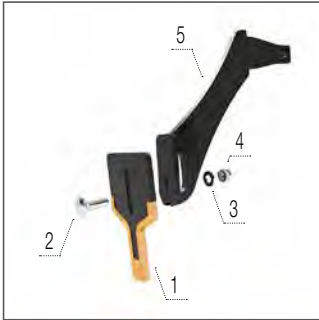
Скребок котка Cutpack з твердосплавним напilenням
