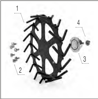
Кільцевий коток 350×100
