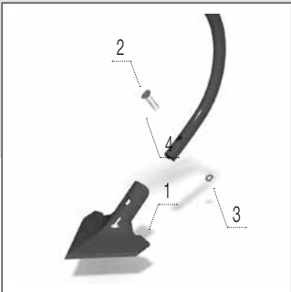
Лапа 150 мм
