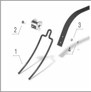
Стійка борони за сошником сівалки
