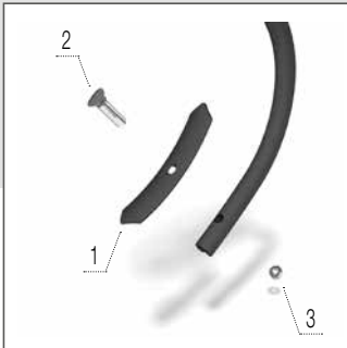
Долото 40 мм
