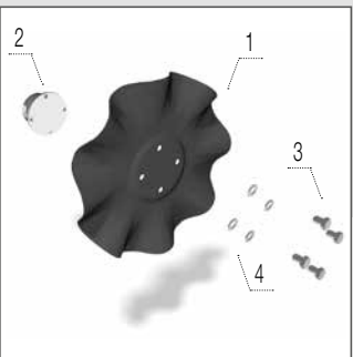
Сошник
