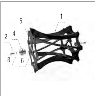
Решітчастий коток 350
