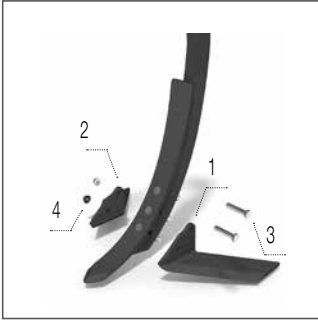
Крила долота 185 мм
