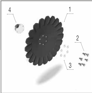
А-диск 460 × 5 мм
