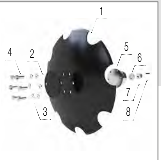
Зубчастий диск 560 × 5 мм
