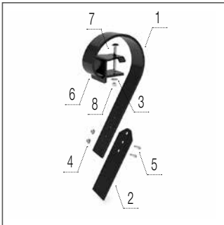
Планка для вирівнювання ґрунту перед подвійним котком
