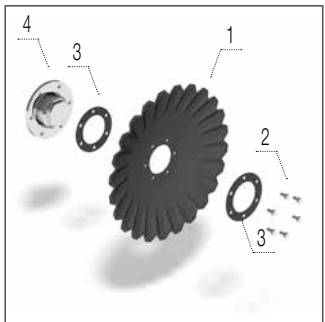
А-диск для центрального вузла 620 × 6 мм
