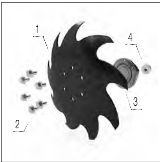
9-RH зірочка
