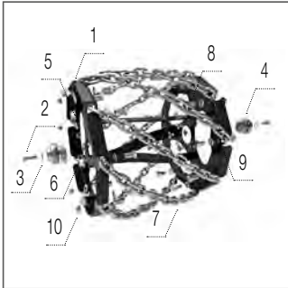
Ланцюговий коток 350
