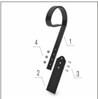
Захист котка
