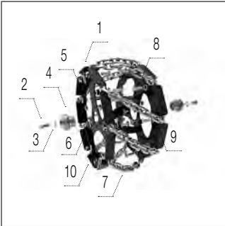
Ланцюговий коток 200
