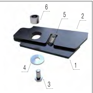
Ножовий скребок
