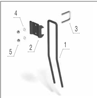
Стійка борони перед одинарним котком
