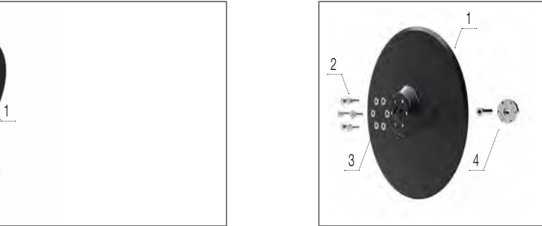
Колесо глибини 330 × 65
