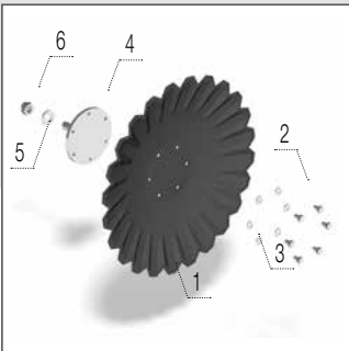
А-диск 620 × 6 мм
