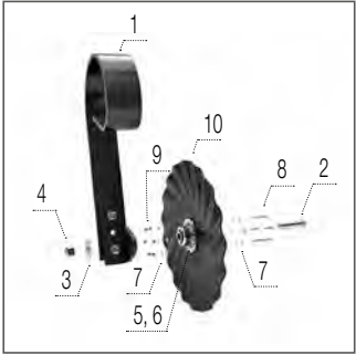
Лівий сошник
