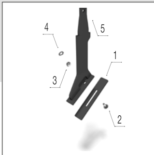
Скребок U-подібного кільцевого котка
