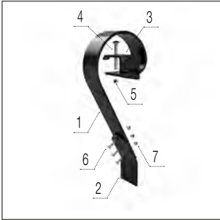
Планка Crushbar – передній вирівнювач
