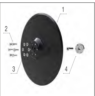
Диск висівного сошника
