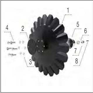
А-диск 560 × 5 мм
