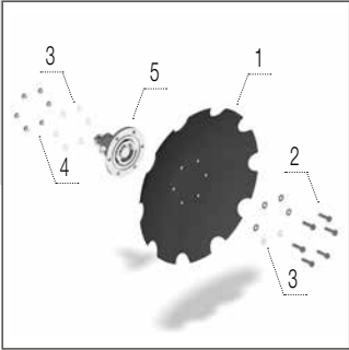
Зубчастий диск 660 × 6 мм
