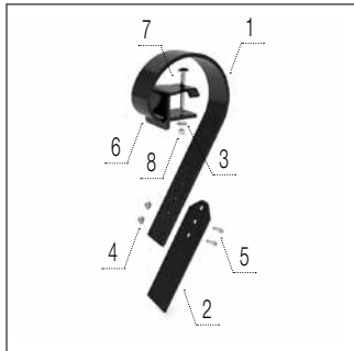
Планка для вирівнювання ґрунту перед одинарним котком
