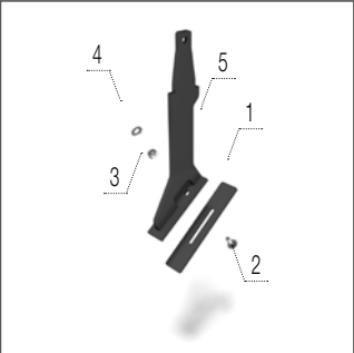
Скребок V-подібного кільцевого катка
