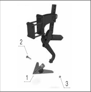
Лапа Слідорозрихлювача
