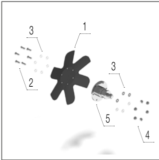
Вирівнювальний зубчастий диск – правий
