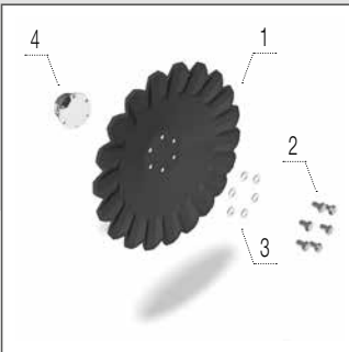
A-диск 460 × 5 мм
