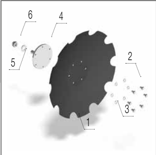
Зубчастий диск 620 × 6 мм
