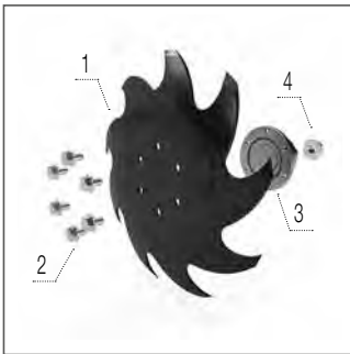
9-LH зірочка
