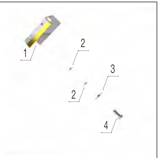
Скребок сошника з твердосплавною накладкою
