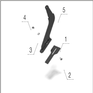
Скребок V-подібного катка
