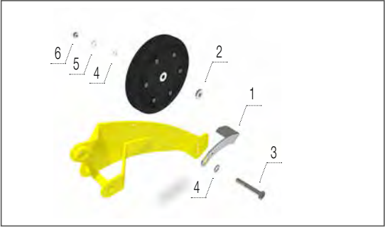
Скребок класичного копіювального колеса
