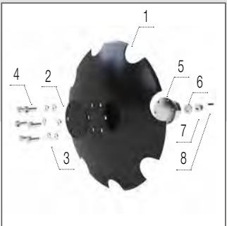
Зубчастий диск 520 × 5 мм
