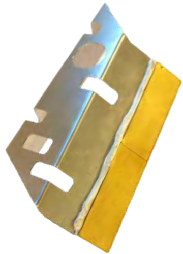
OMEGA OO_L, OO_FL KM060563 Скребок сошника (1 шт)
