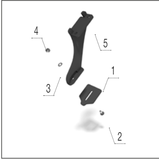
Скребок котка Cutpack
