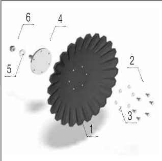
А-диск 620 × 6 мм
