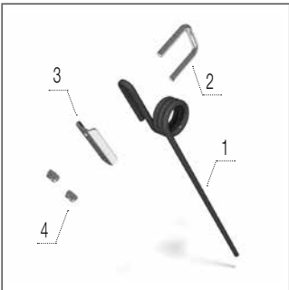
Стійка борони 10 mm
