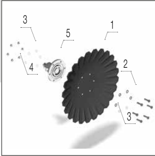
А-диск 660 × 6 мм
