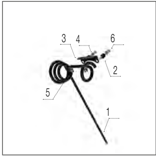
Ліва трирядна стійка борони
