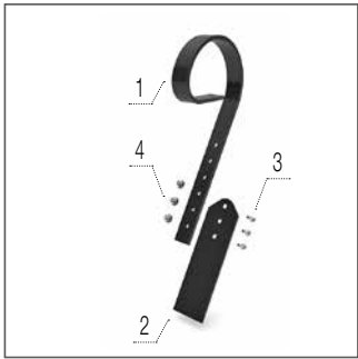
Захист котка під важелем котка
