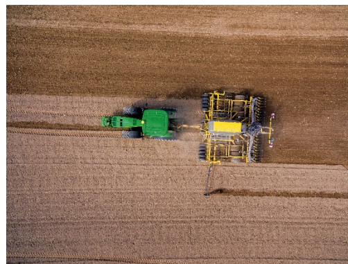
Diskové sekce jsou navrženy do tvaru „X“, což zajišťuje přesné držení stopy za traktorem
