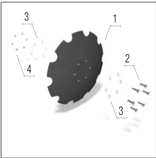
Disco dentado 690 x 6 mm
