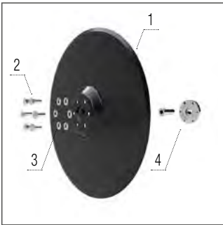
Disco de siembra
