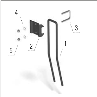
Rastrillas delanteras
