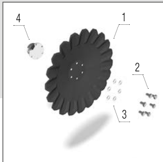
Disco A 520 x 5 mm
