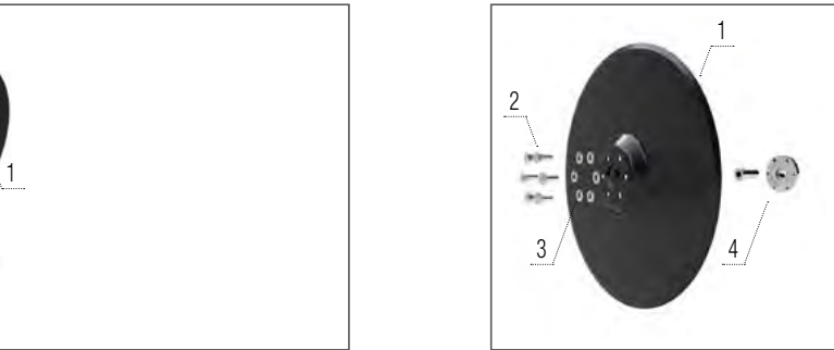
Rueda de profundidad 330 × 65
