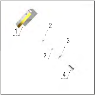
Rasgadores de disco de siembra de carburo
