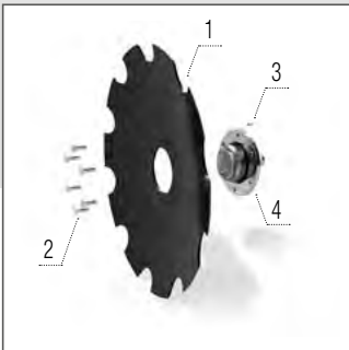
Disco dentado en unidad central 620 × 6 mm
