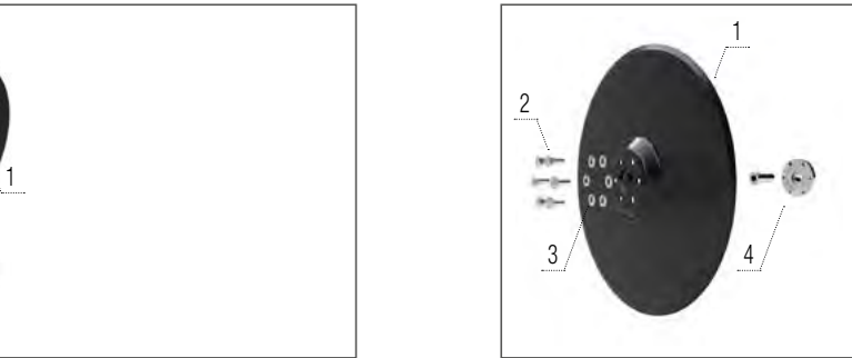
Rueda de profundidad 330 x 65
