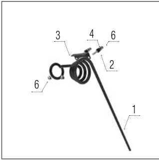
Rastrillas de tres hileras derecha
