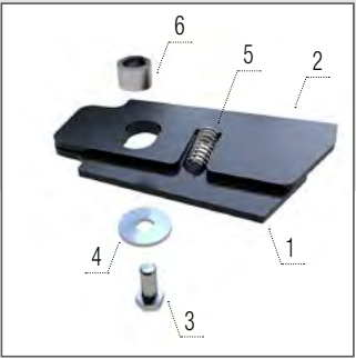
Rasgadores de tijera
