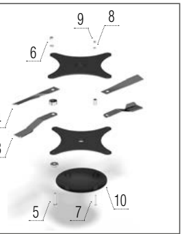
Cuchillas de maíz – derecha + cubierta del rotor
