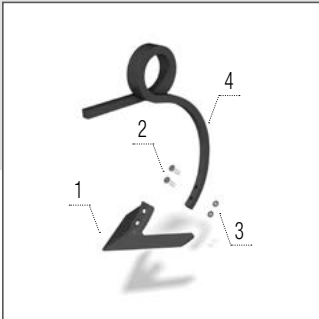
Reja – derecha
