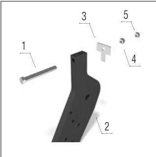
Tornillo de arrastre D
