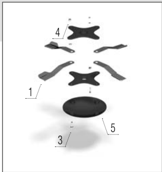
Cuchillas de hierba – izquierda + tapa del rotor
