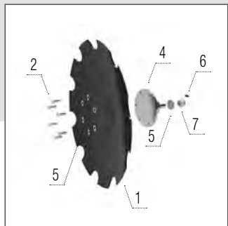
Disco dentado 620 × 6 mm
