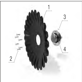
Disco A a unidad central 620 × 6 mm
