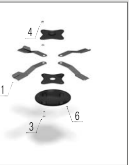
Cuchillas de hierba – centro + tapa del rotor
