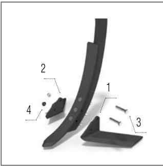
Cinzel alas 185 mm
