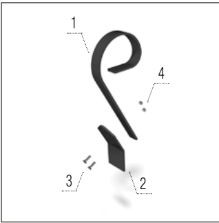
Pala Crushbar
