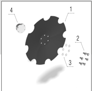
Disco dentado 460 x 5 mm
