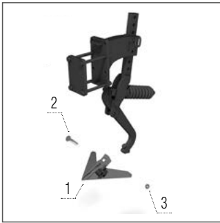
Reja cultivadora stop
