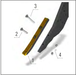
Cinzel 40 mm LONG LIFE
