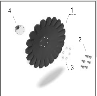
Disco A 460 x 5 mm
