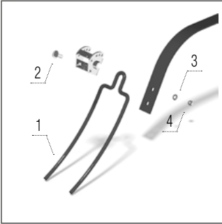
Rasrta cubresemillas detrás del disco de siembra
