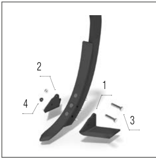
Cinzel alas 125 mm
