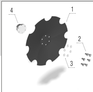
Disco dentado 520 x 5 mm
