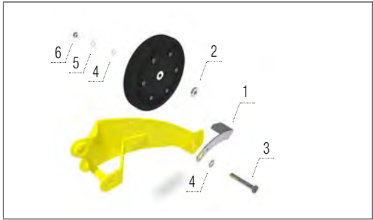
Rasgadores de rueda de profundidad Classic
