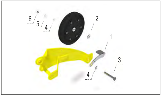
Rasgadores de rueda de profundidad Hardface
