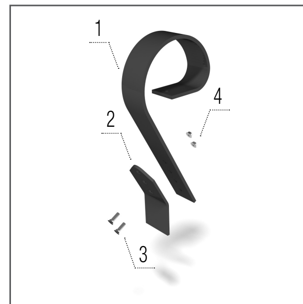
Paddle Crushbar
