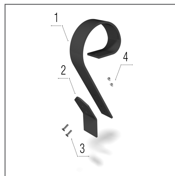
Lopatka Crushbar
