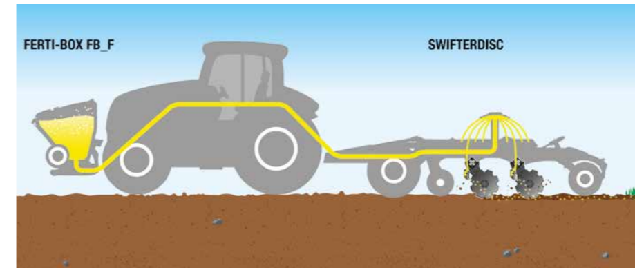
5. Možnost propojení předního nebo zadního FERTI-BOXU s diskovými podmiťáči SWIFTERDISC
