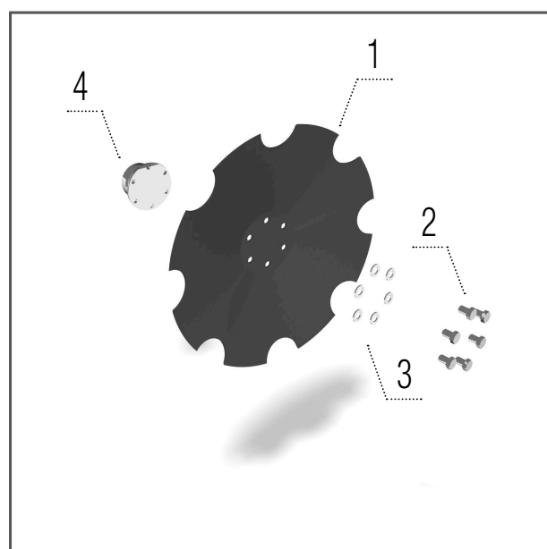
Зубчатый диск 520 × 5 мм
