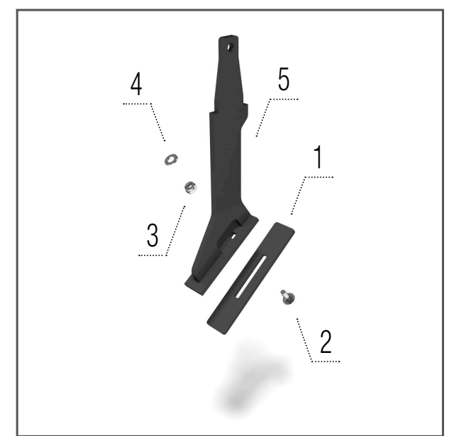
Чистики V-ring каток
