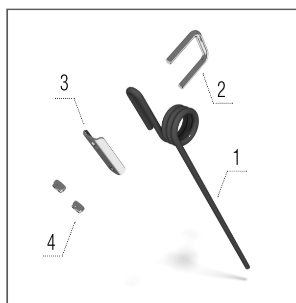
Peignes de herse 10 mm
