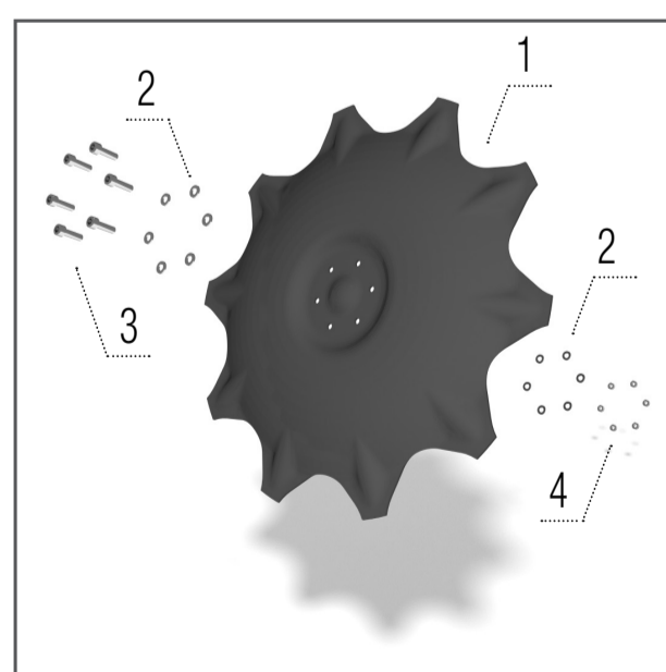
Disque de protection
