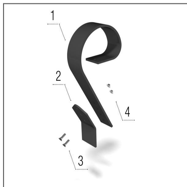
Paddle Crushbar
