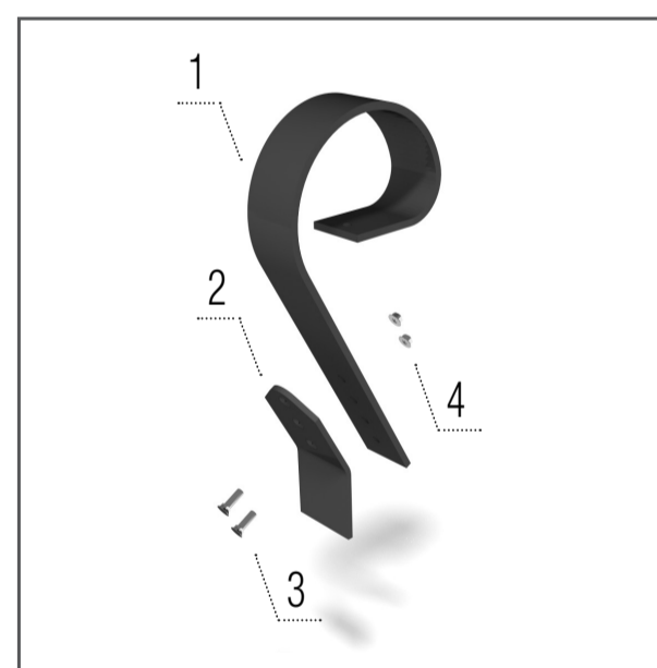
Paddle Crushbar
